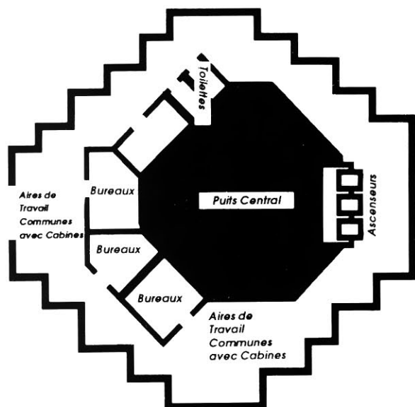
PLAN D'UN ETAGE TYPE
