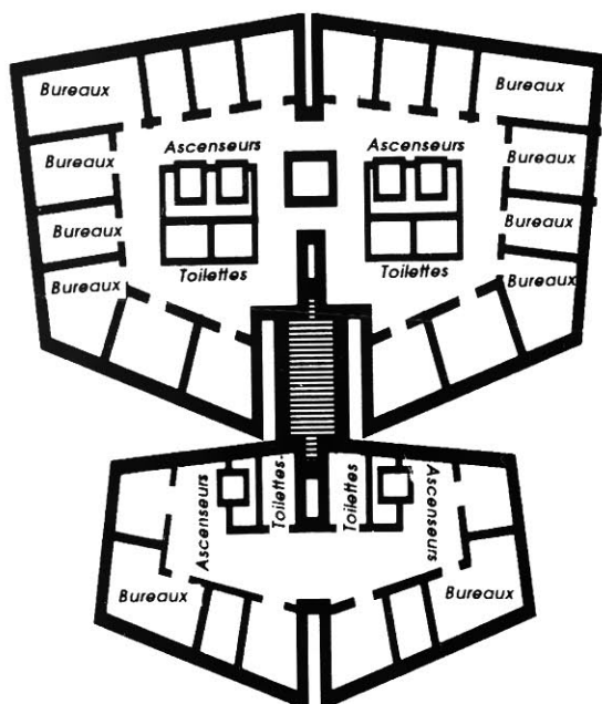
PLAN D'UN ETAGE TYPE
