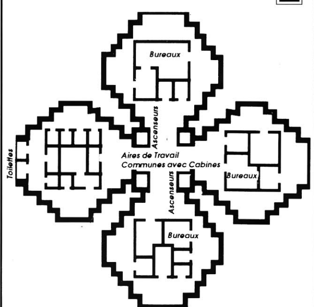
PLAN D'UN ETAGE TYPE
